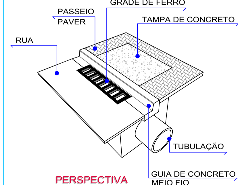
PERSPECTIVA
