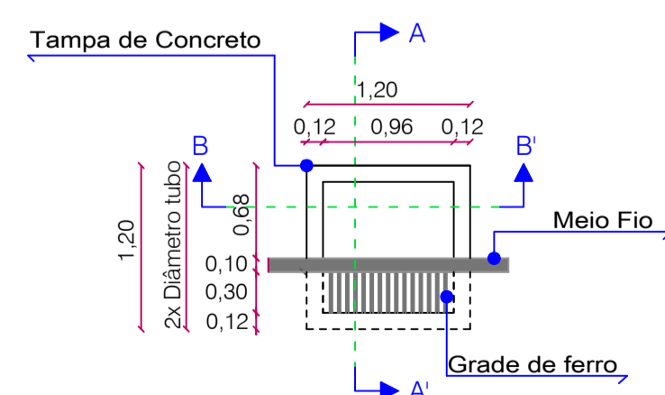
VISTA SUPERIOR
