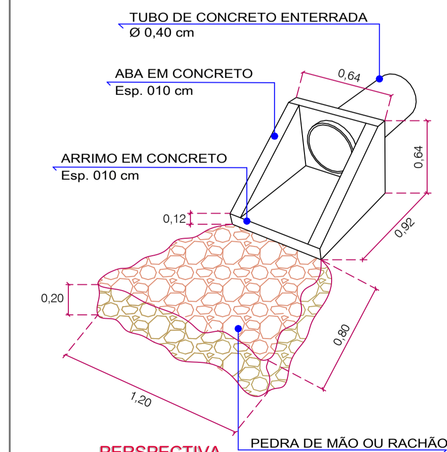
PERSPECTIVA
