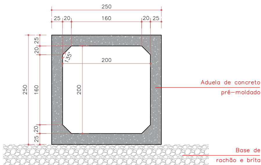
DETALHE ADUELA 2x2 - ELEVACÃO ESC. 1:50
