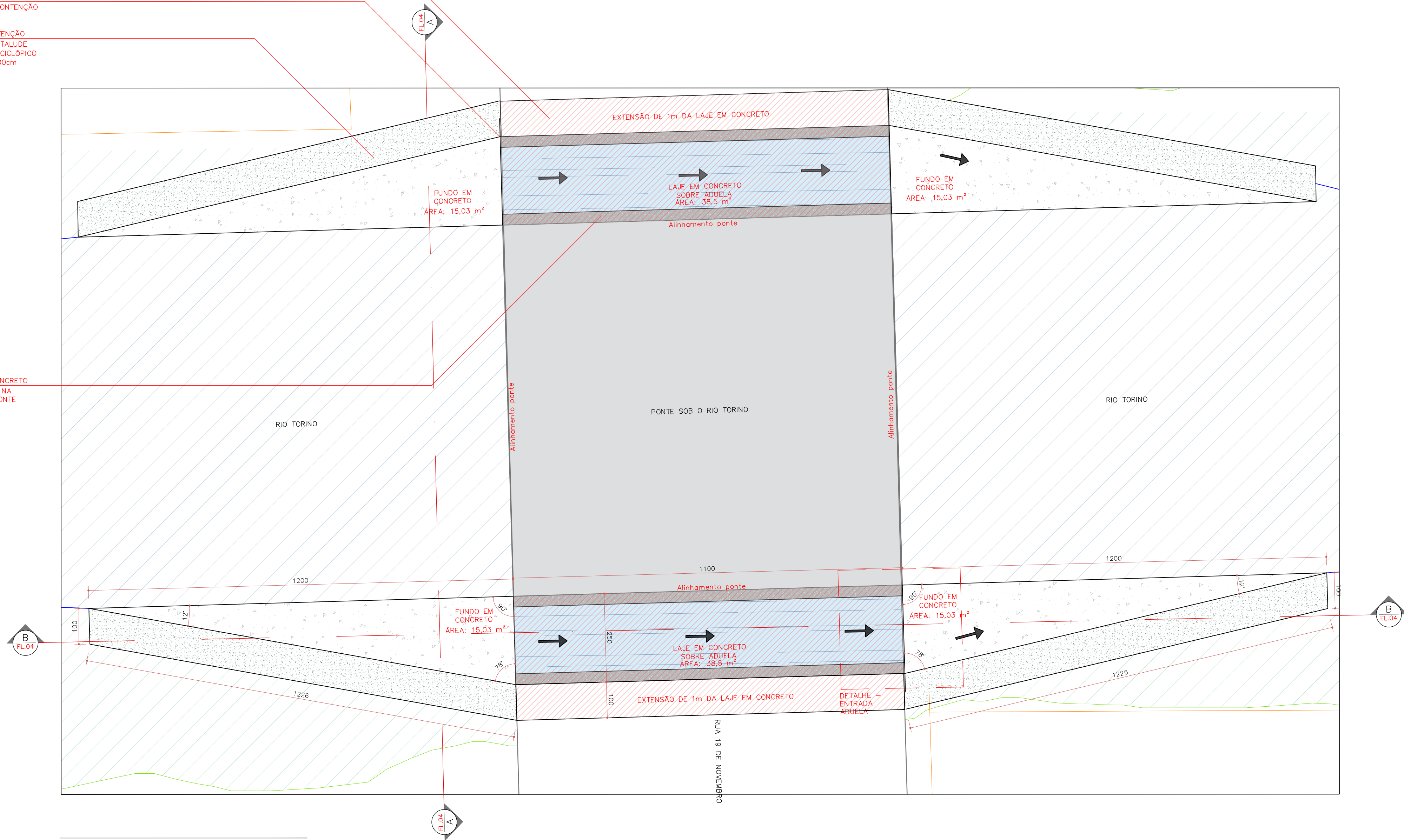
PLANTA BAIXA — CANAL JUSANTE ESC. 1:75
