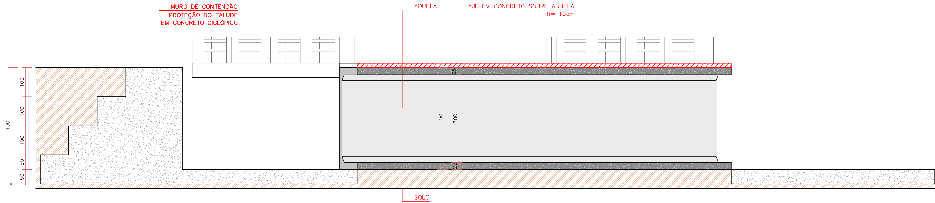
CORTE A-A – CANAL JUSANTE ESC. 1:75
