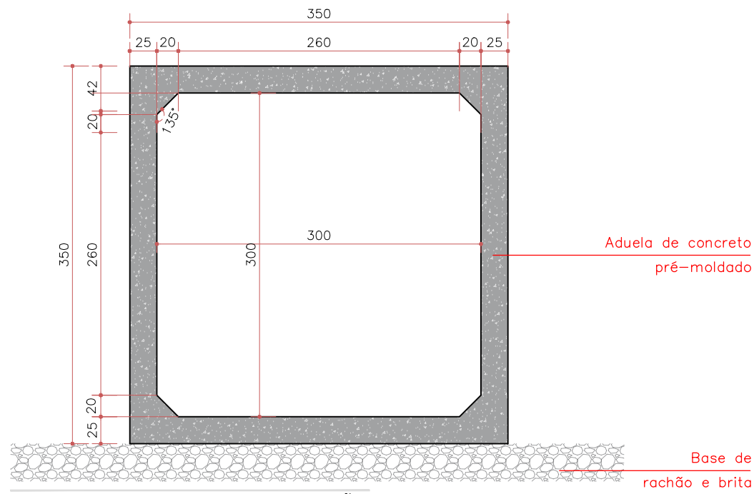
DETALHE ADUELA 3x3 – ELEVÇÃO ESC. 1:50
