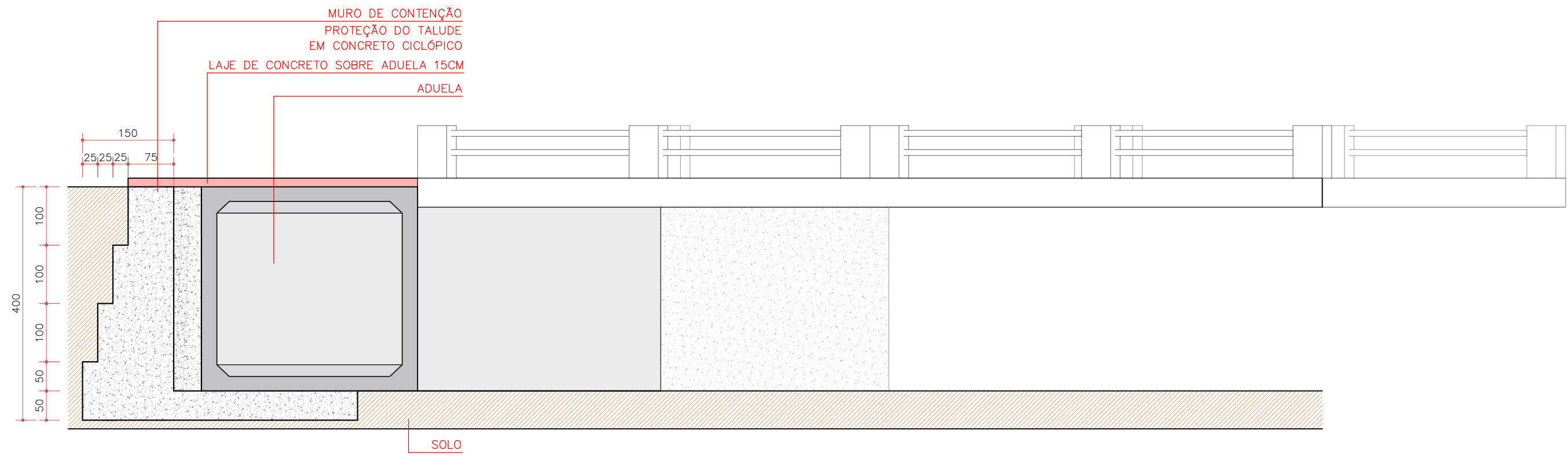
CORTE B-B – CANAL JUSANTE ESC. 1:75
