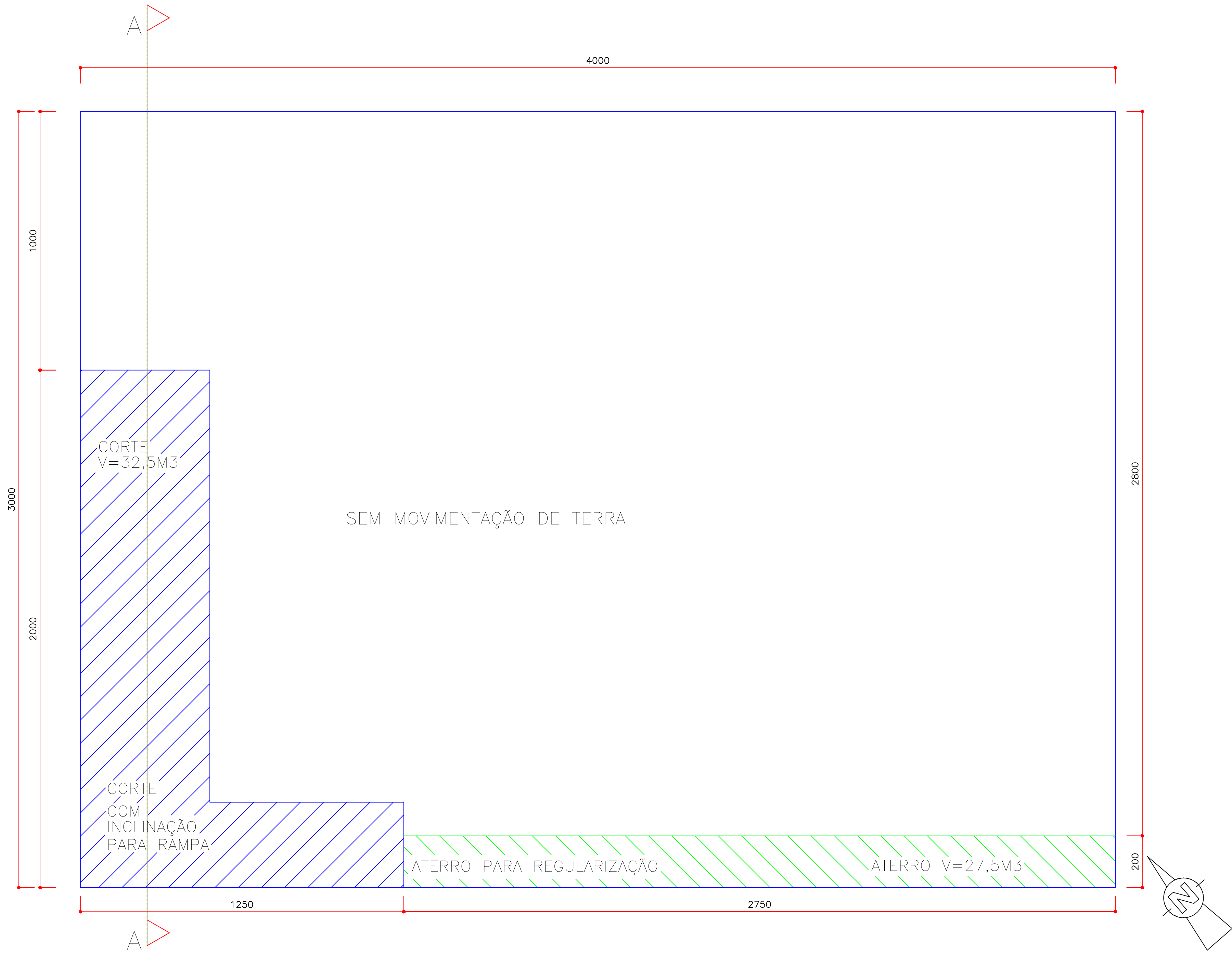
PLANTA CORTE E ATERRO ESC. 1:100
