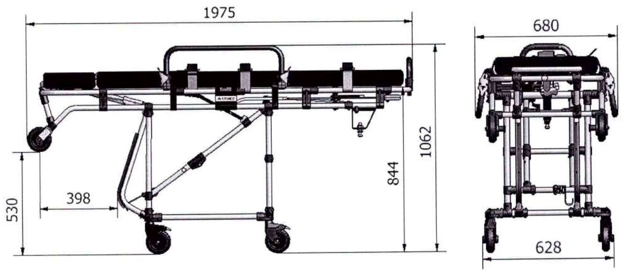
Figura 02 – Maca Armada
