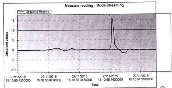
Figura 07 – Aceleração frontal
