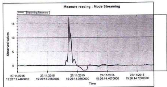
Figura 03 – Aceleração vertical
