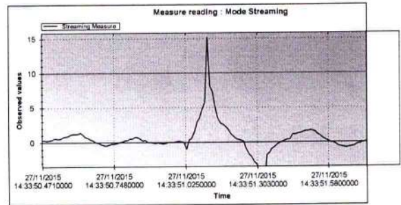
Figura 05 – Aceleração lateral
