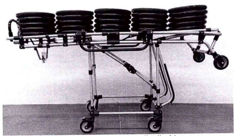
Figura 05 - 500 kg de carga distribuída
