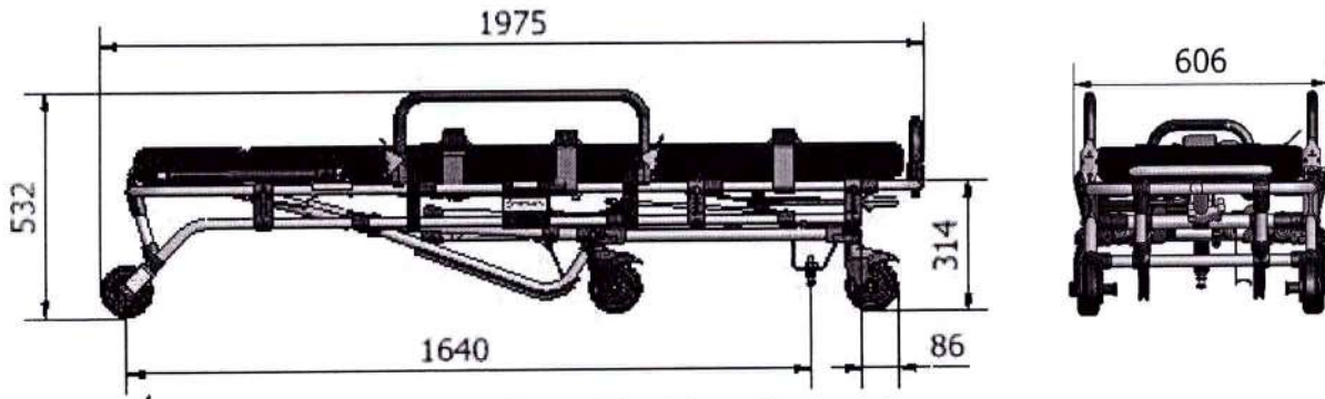
Figura 03 – Maca desarmada
