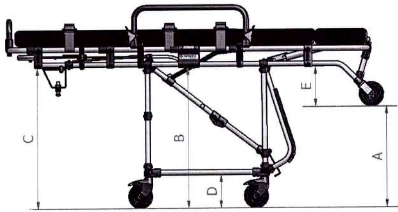
Figura 04 - Vista lateral
