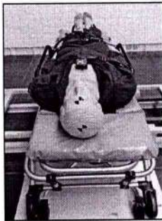
Figura 04 – Impacto lateral (depois do teste)
