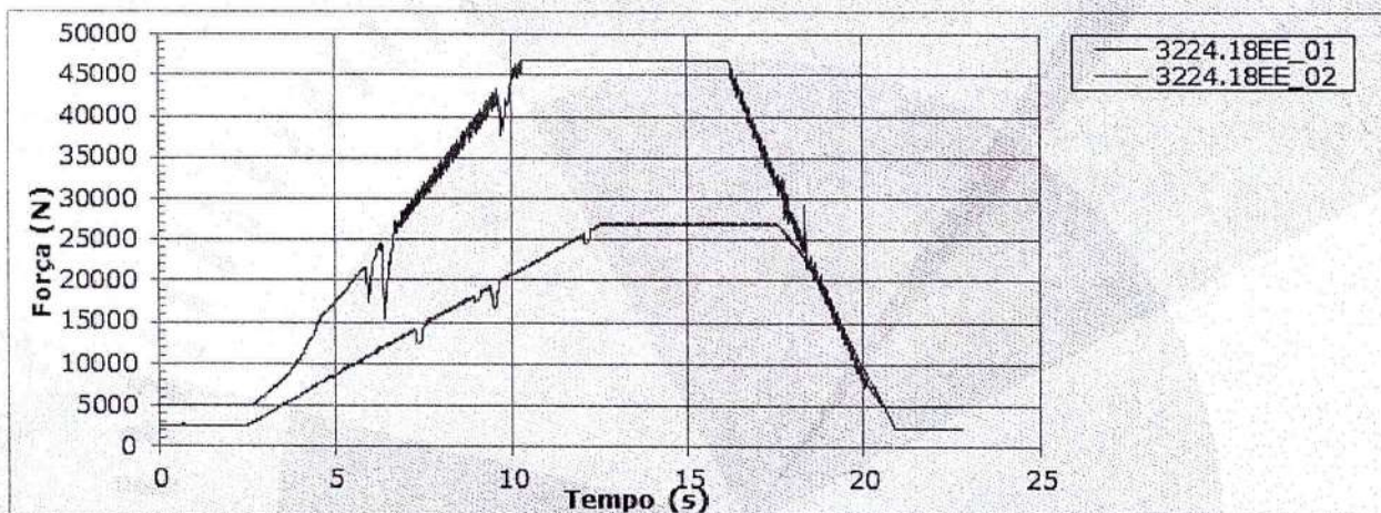
Figura 3: Gráfico Força (N) x Tempo (s).
