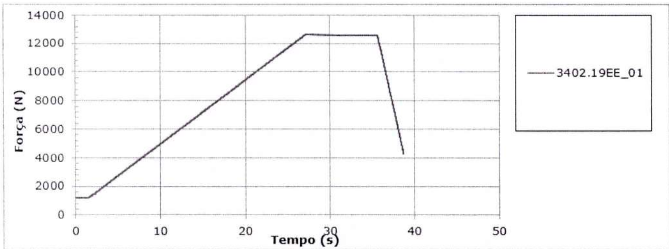
Figura 3: Gráfico Força (N) x Tempo (s).
