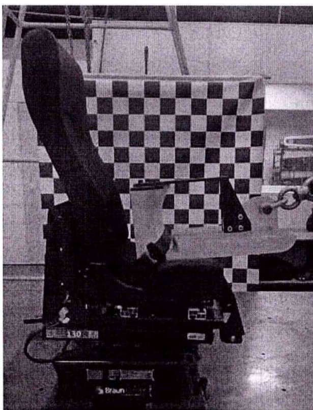
Figura 1: Foto da configuração de ensaio.
