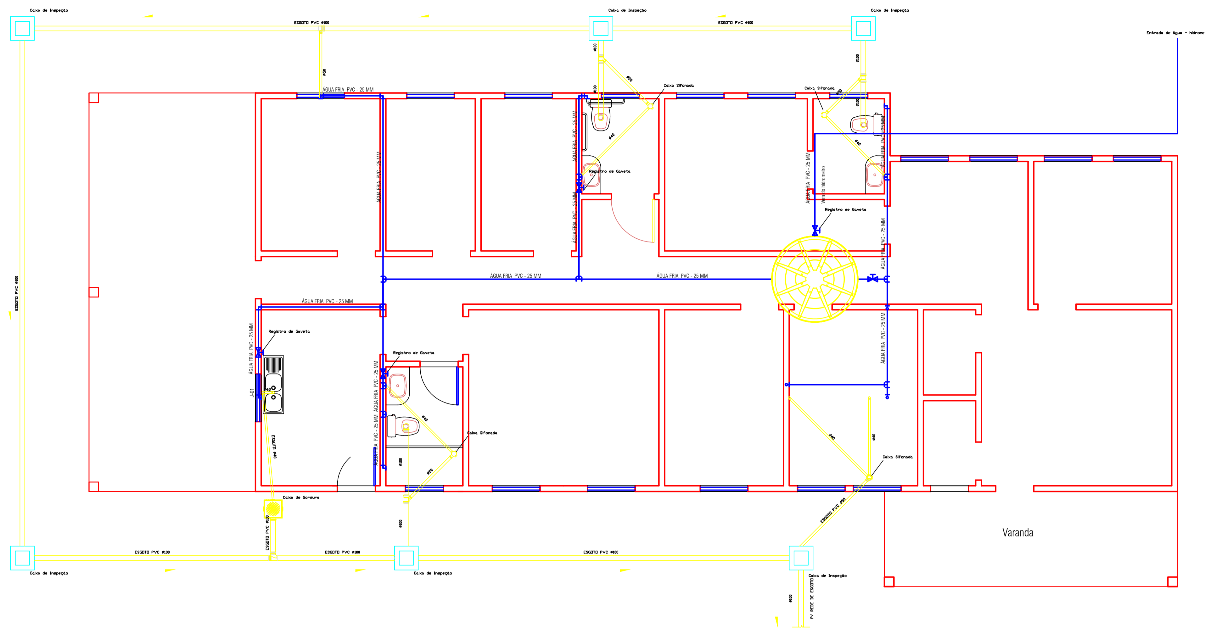
PLANTA BAIXA Área Total - 149,57 m 2 Escala 1:50
