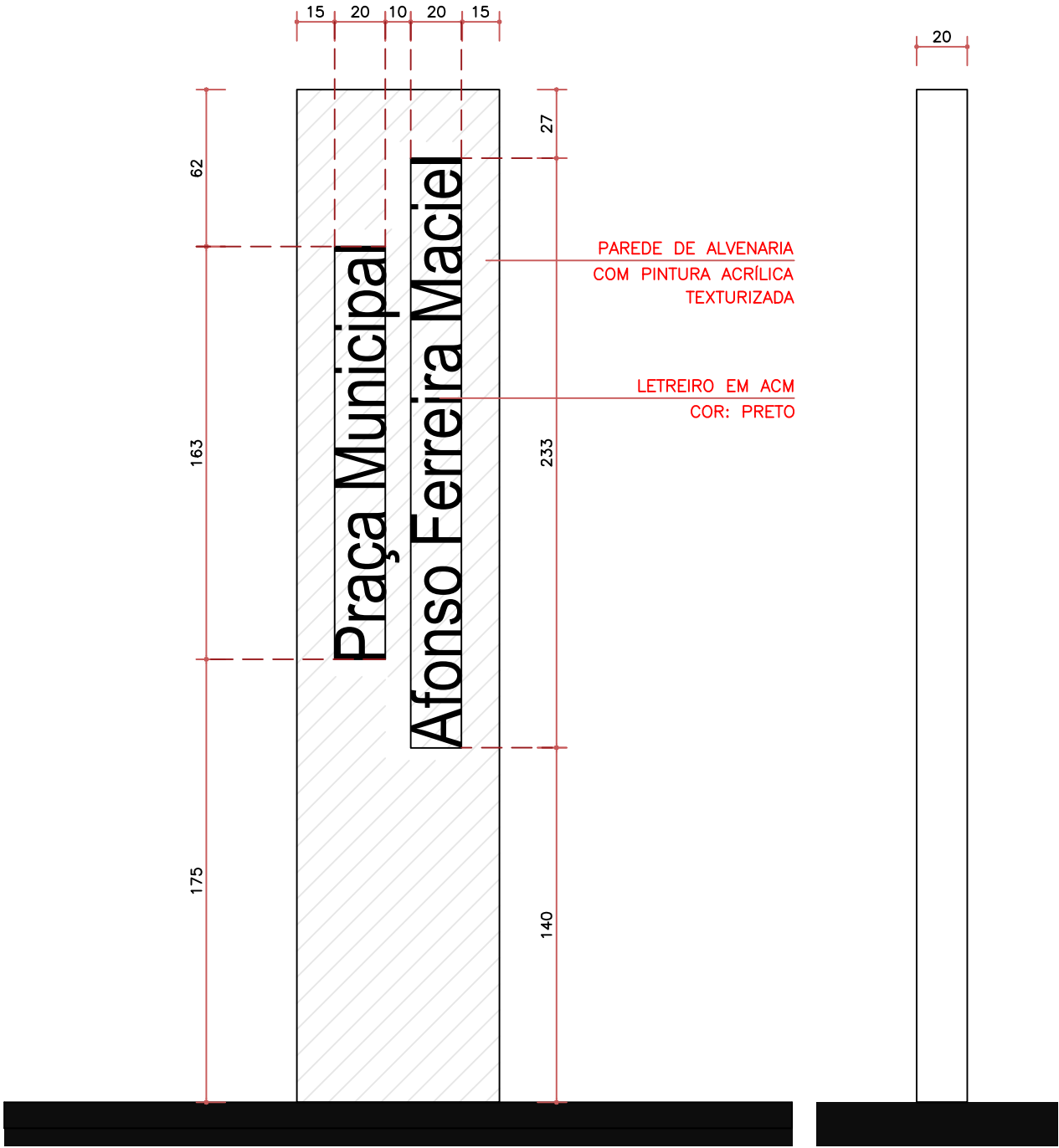
VISTA FRONTAL – PAREDE NA PRAÇA AFONSO FERREIRA MACIEL ESC. 1:25
