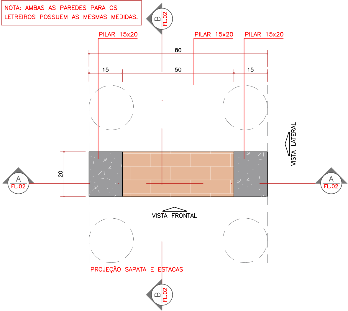
PAREDE DE ALVENARIA PARA LETREIRO – PLANTA BAIXA ESC. 1:10
