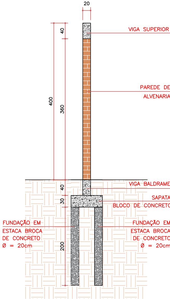
CORTE B-B ESC. 1:25
