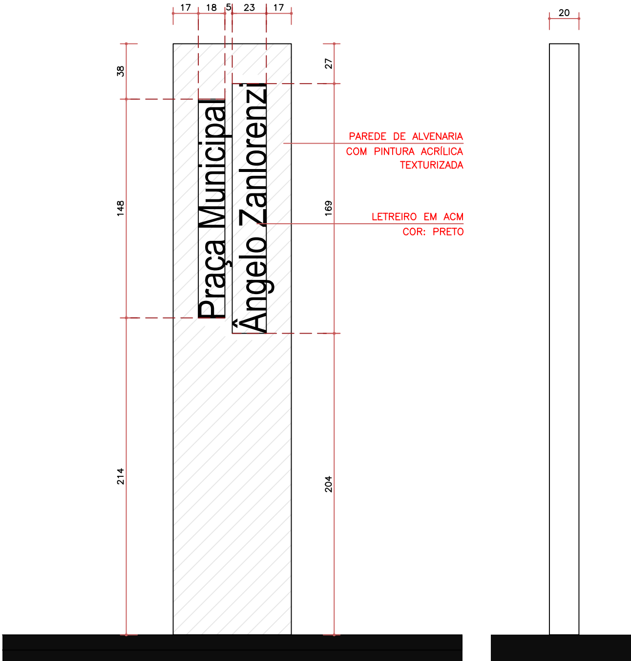
VISTA FRONTAL – PAREDE NA PRAÇA ÂNGELO ZANLORENZI ESC. 1:25
