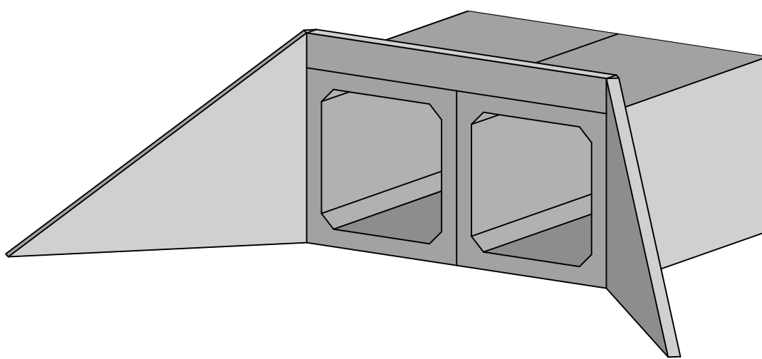
DETALHE 01 - ENTRADA ADUELAS - ISOMÉTRICA ESC. 1:75
