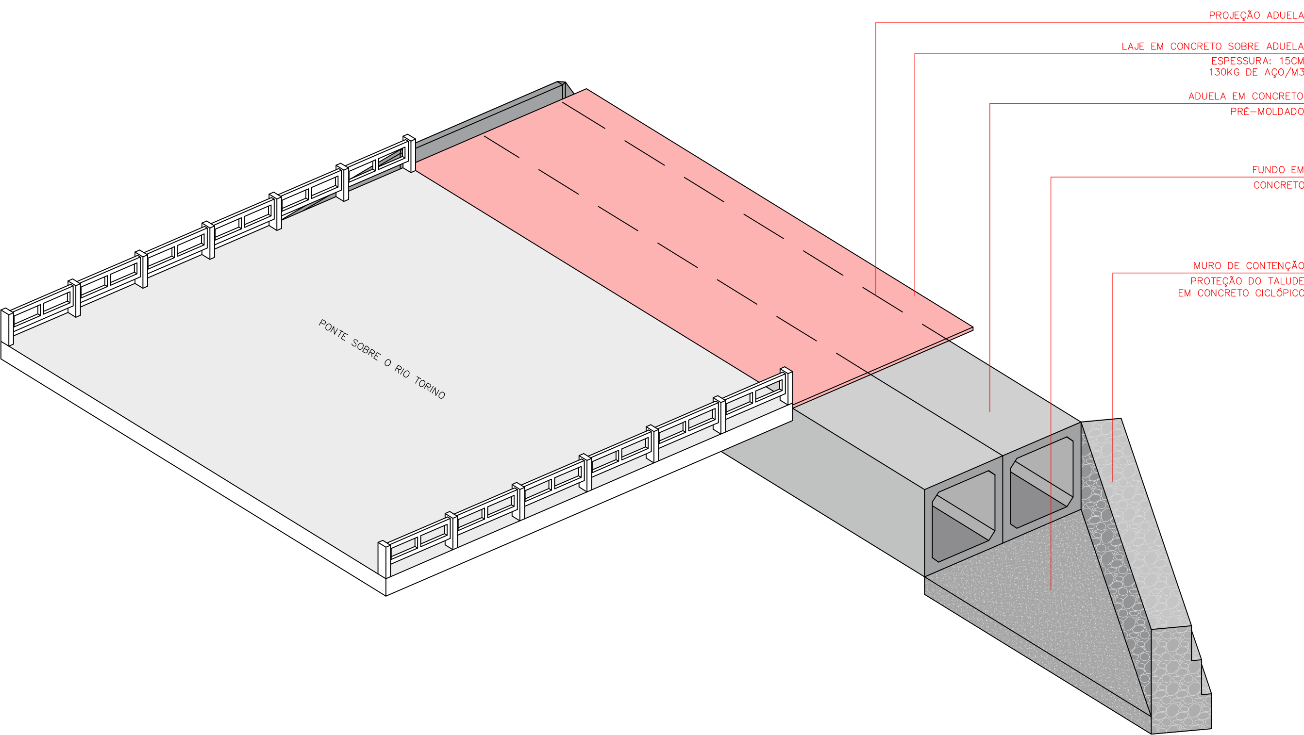
PERSPECTIVAS ISOMÉTRICAS ESC. S/E
