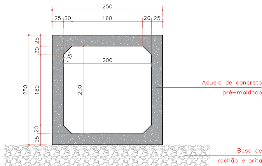
DETALHE ADUELA 2x2 - ELEVÇÃO ESC. 1:50
