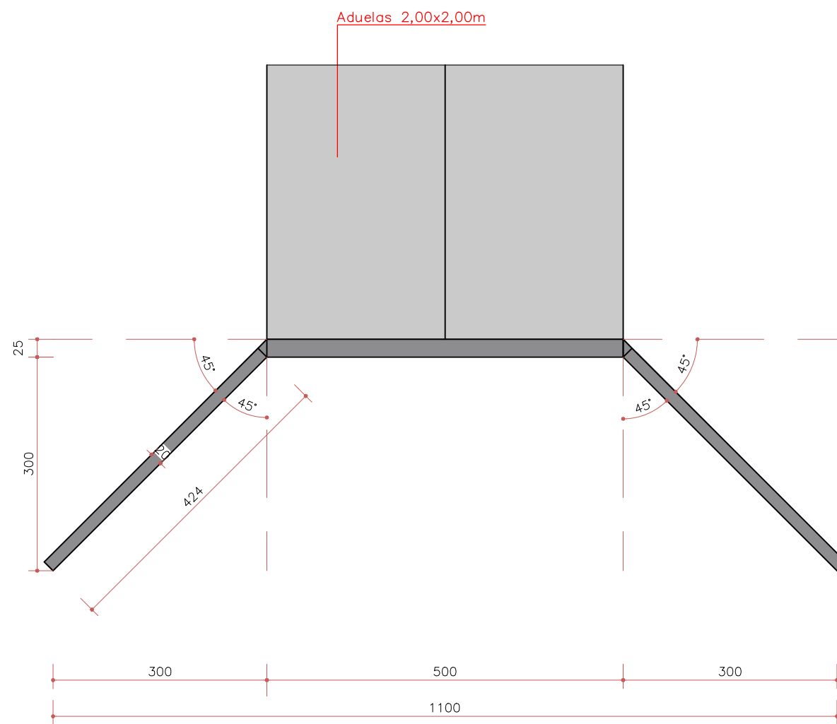
DETALHE 01 - ENTRADA ADUELAS - PLANTA BAIXA ESC. 1:75
