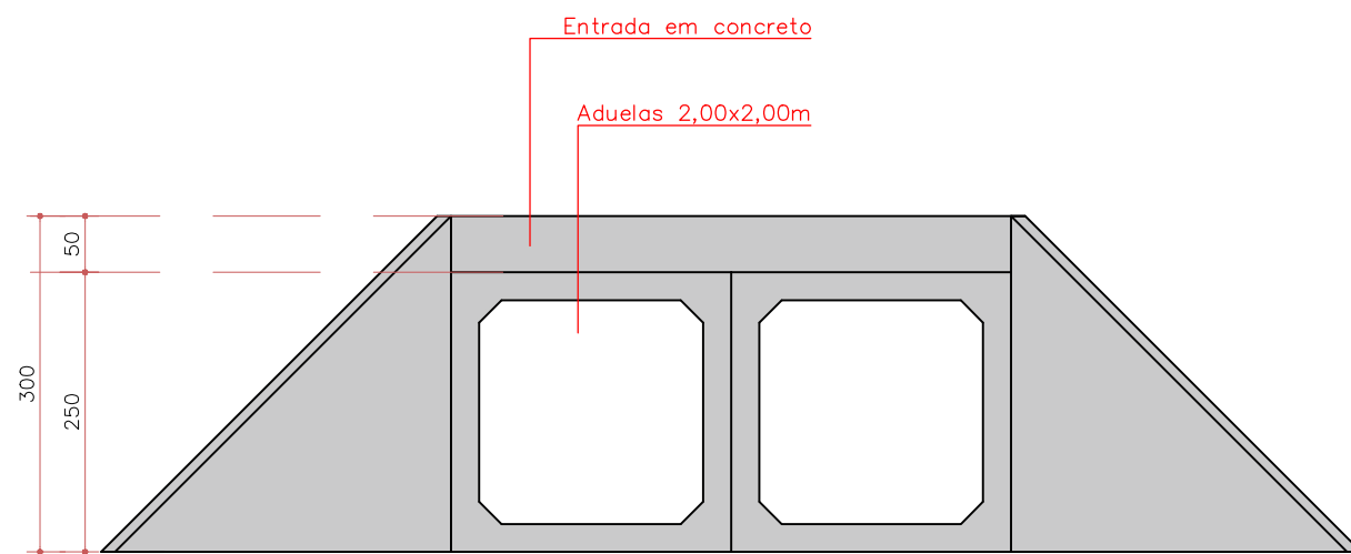
DETALHE 01 - ENTRADA ADUELAS - VISTA FRONTAL ESC. 1:75
