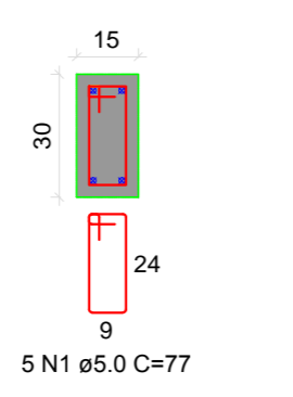
DETALHE DO PILAR 04 ESC 1:20
