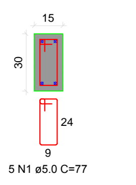
DETALHE DO PILAR 01 ESC 1:20
