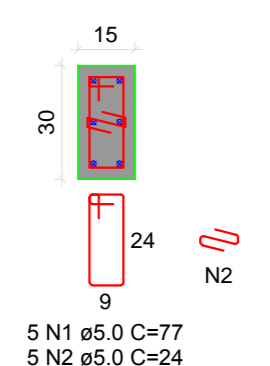
DETALHE DO PILAR 02 ESC 1:20
