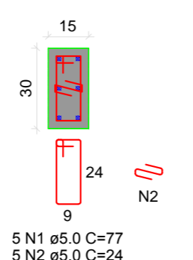
DETALHE DO PILAR 05 ESC 1:20
