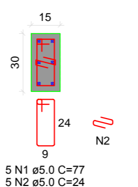
DETALHE DO PILAR 06 ESC 1:20
