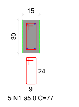
DETALHE DO PILAR 03 ESC 1:20
